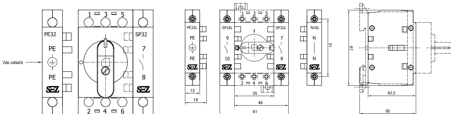
TYP K 32 JD
