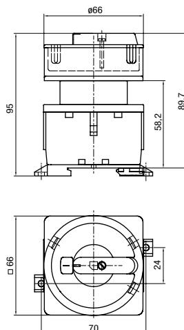
TYP K 32 JLU
