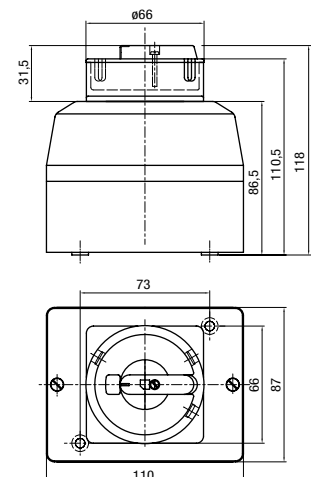
TYP K 32 JPU
