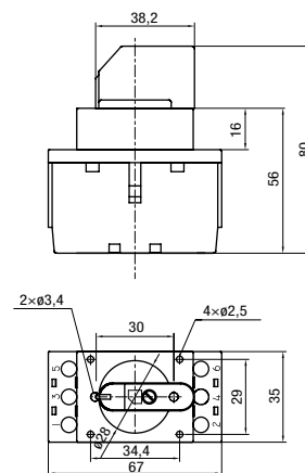
TYP K 32 J
