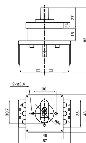
TYP K 32 JDM
