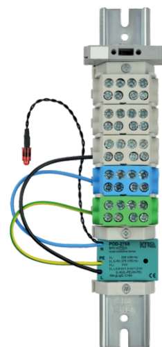
SS POD 516 P TN-S
