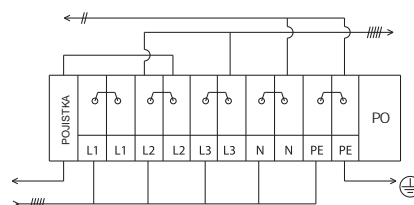
schéma TN-S pr b žné
