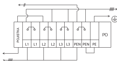
schéma TN-C pr b žné
