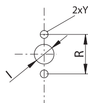
Upevnenie ovládacieho prvku na panel
